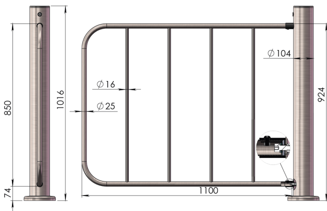
3V Model B со створкой 1100 мм
